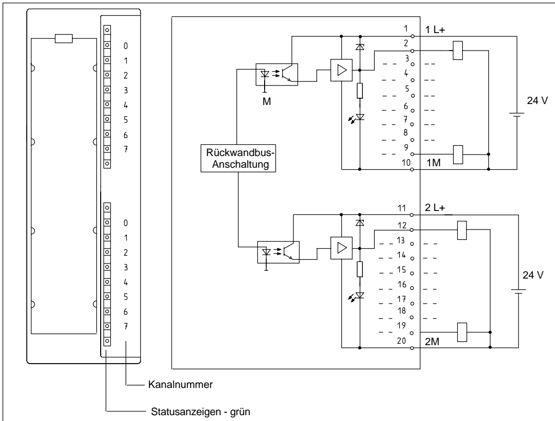
Bild 3-21 Baugruppenansicht und Prinzipschaltbild der SM 322; DO 16 x DC 24 V/0,5 A High Speed
