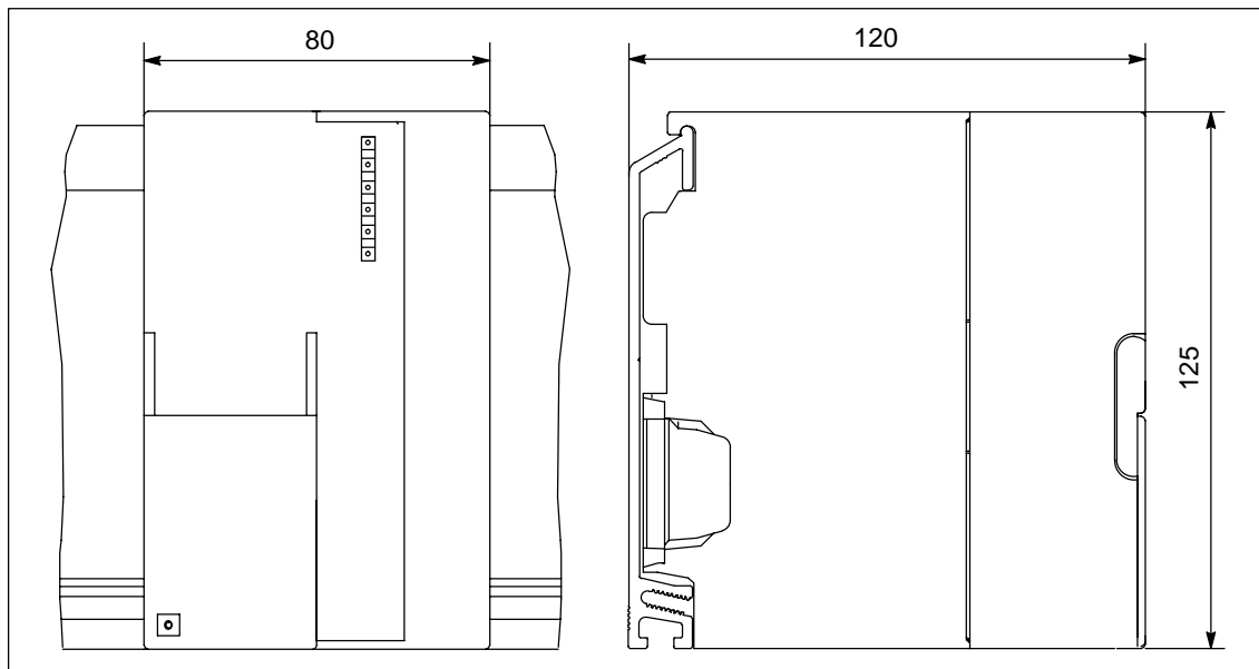
Bild C-18 Anschaltungsbaugruppe IM 361
