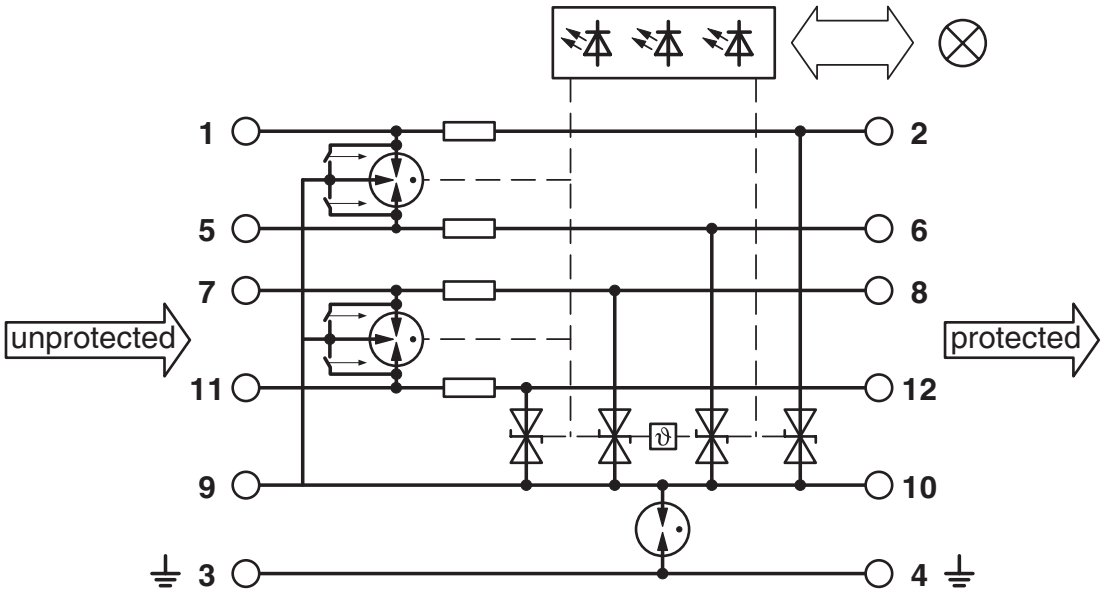
电路图
