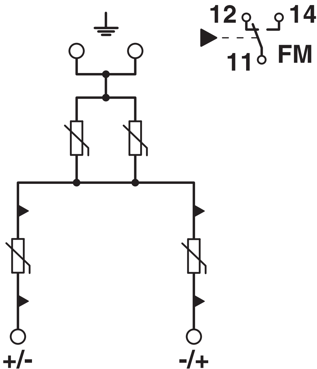
电路图
