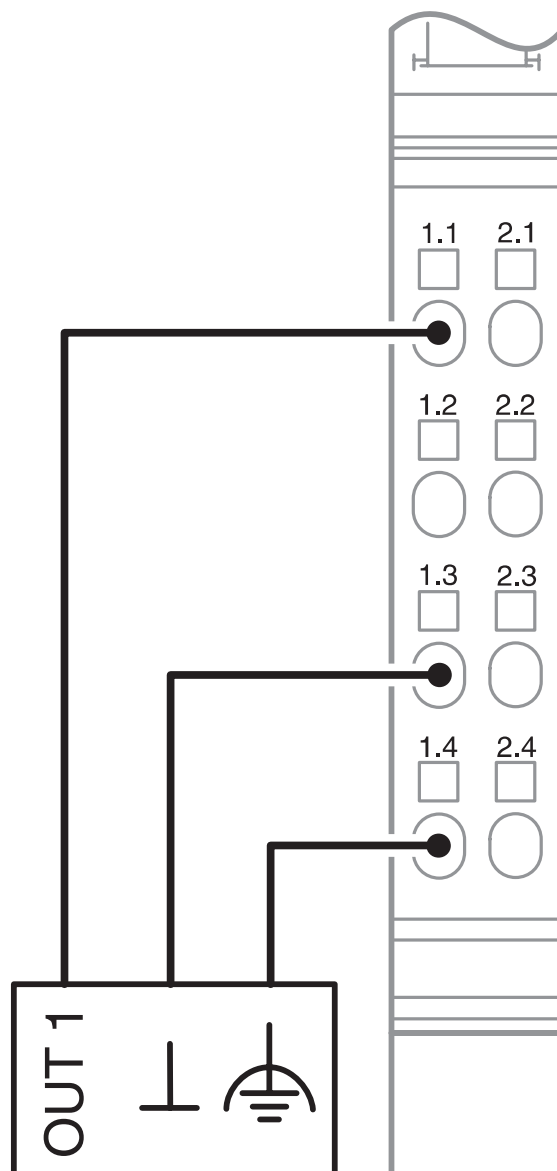
接线图
