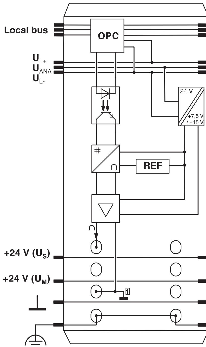
结构框图
