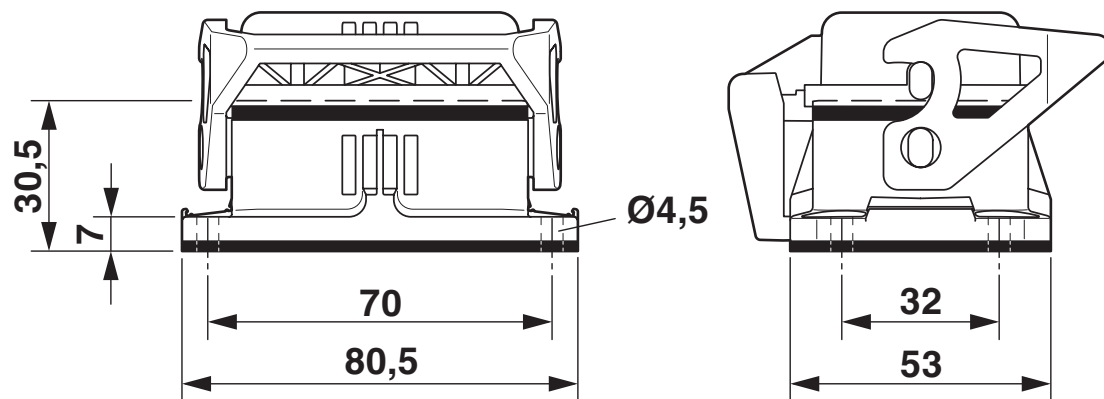
尺寸图
