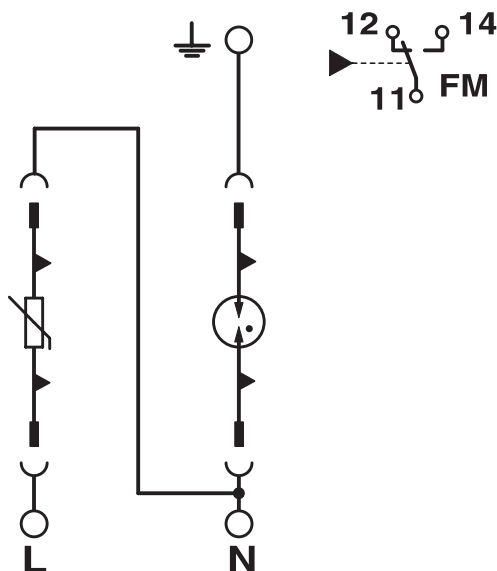
电路图
