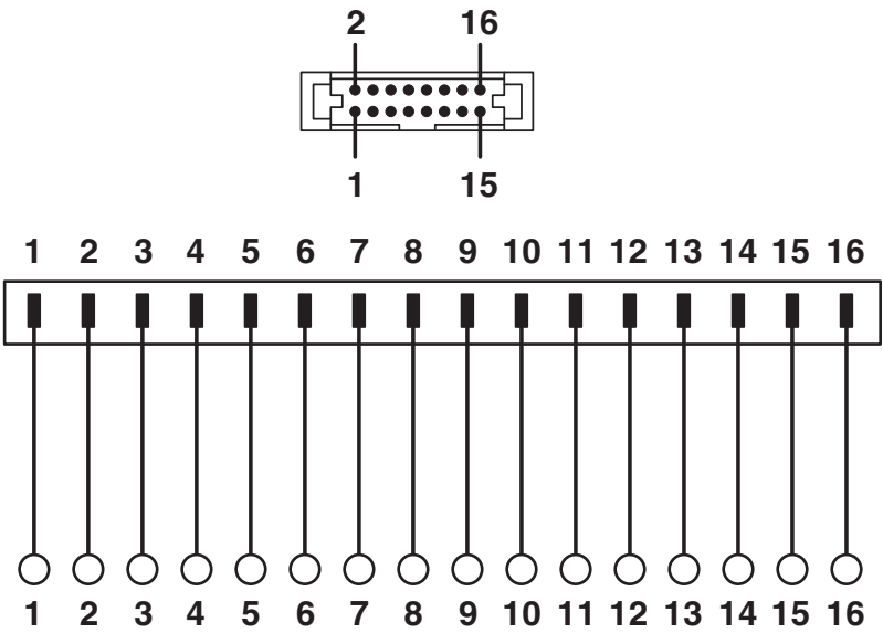
电路图
