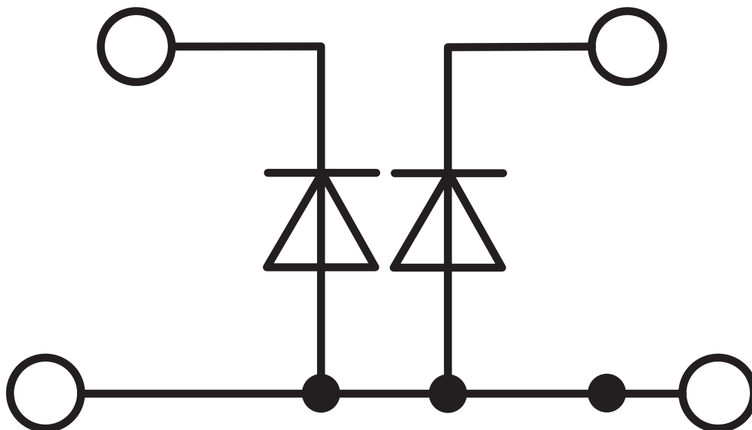
电路图
