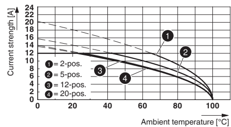
Type: MSTB 2,5/16-STF-5,08 with MSTBV 2,5/16-GF-5,08
