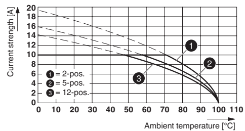
Type: MSTB 2,5/16-STF-5,08 with MDSTBV 2,5/16-GF-5,08
