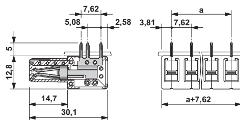
外形寸法
