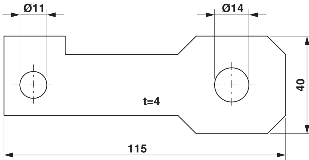
尺寸图
