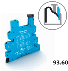
Push-In terminal socket 35 mm rail mounting (EN 60715)
