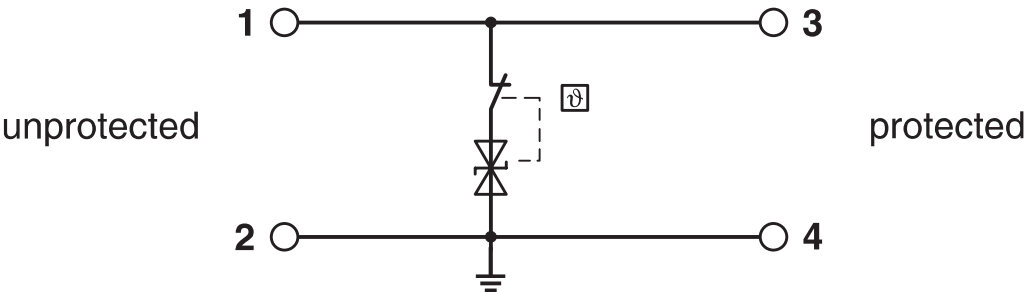
电路图
