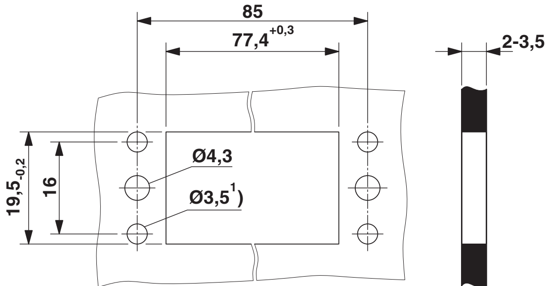
尺寸图
