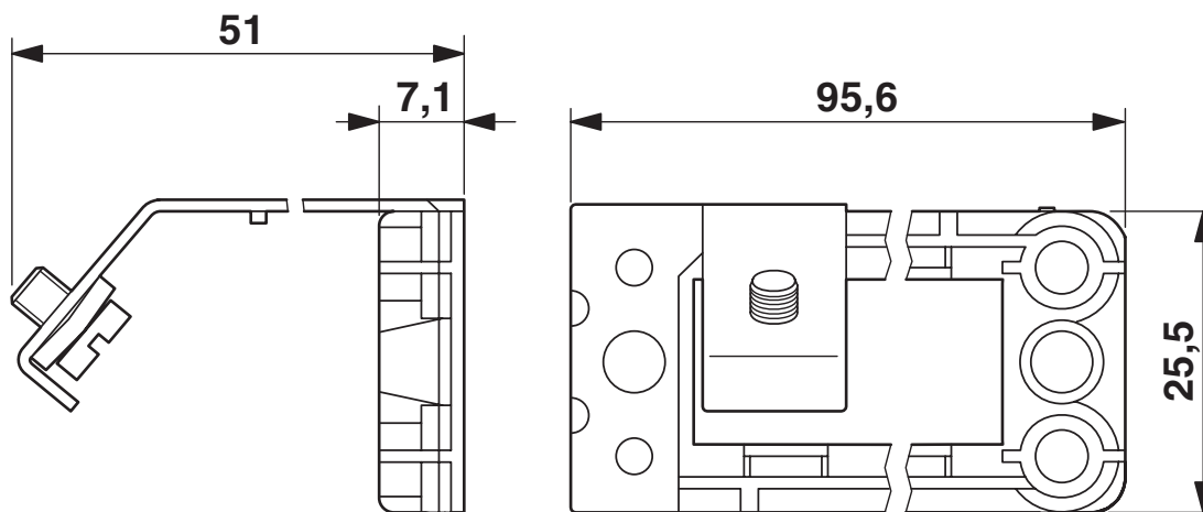
尺寸图
