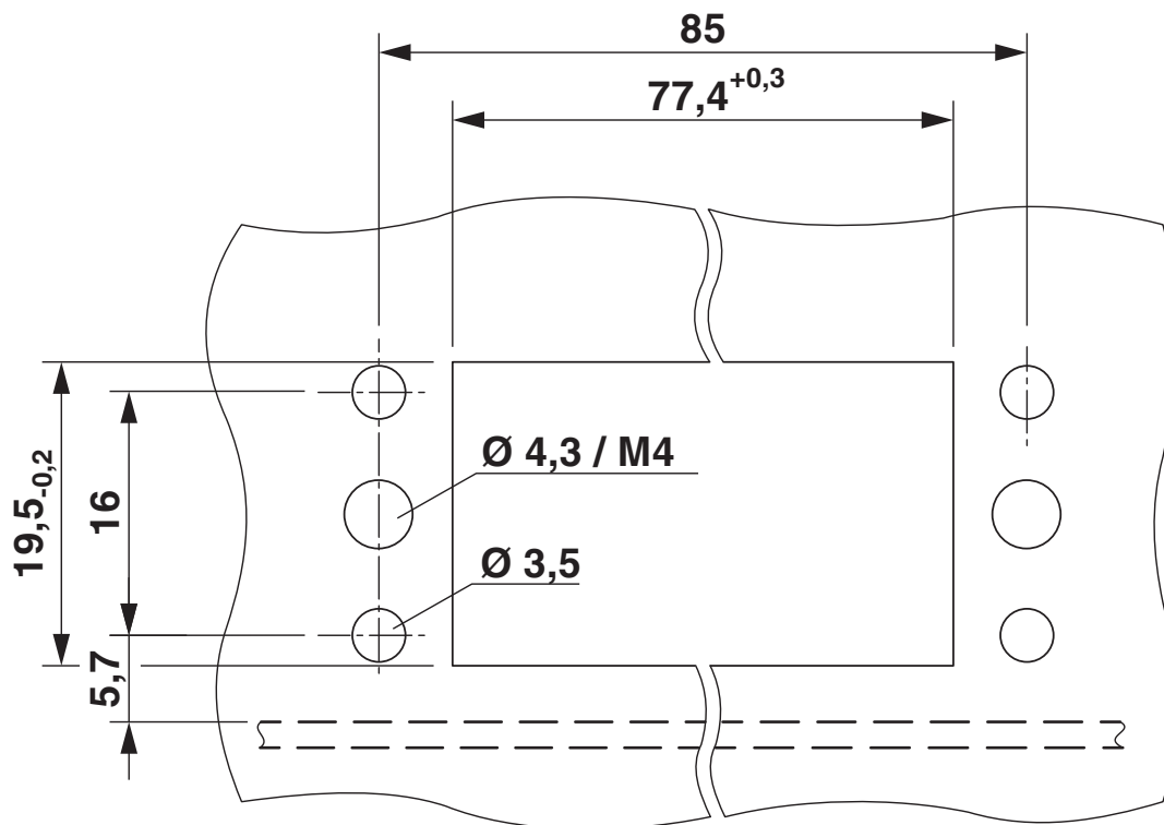
尺寸图
