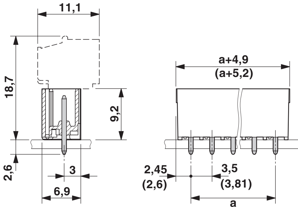
尺寸图
