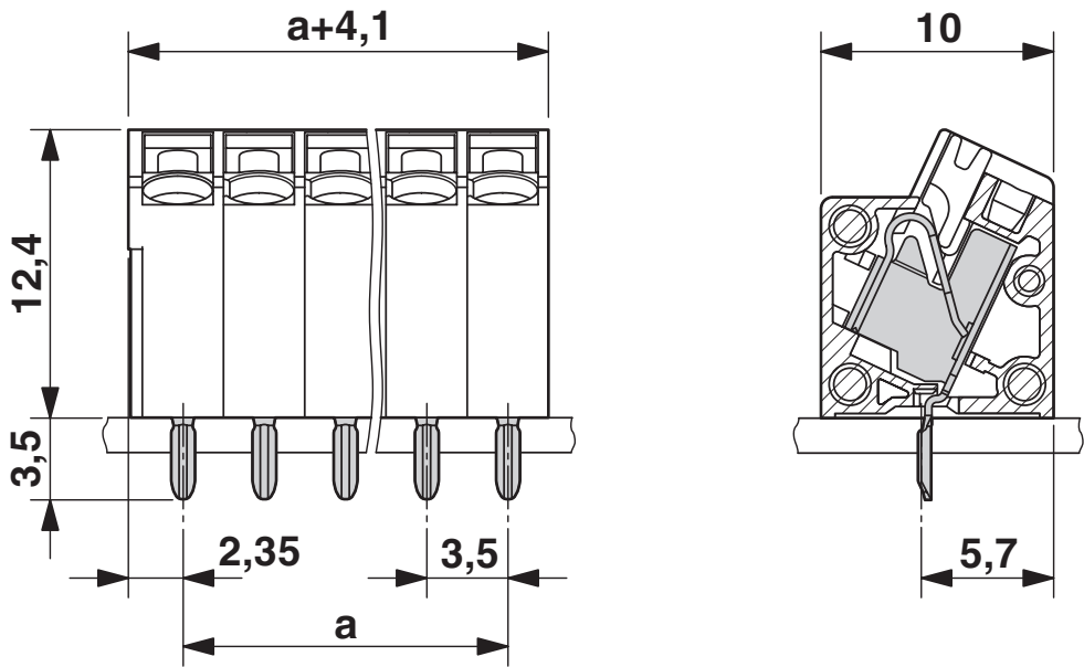
尺寸图
