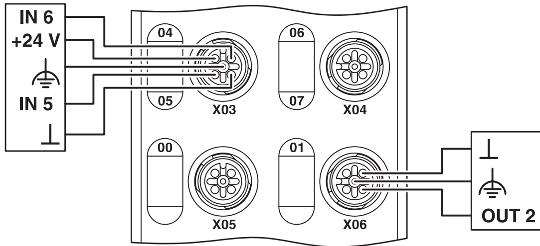
接线图
