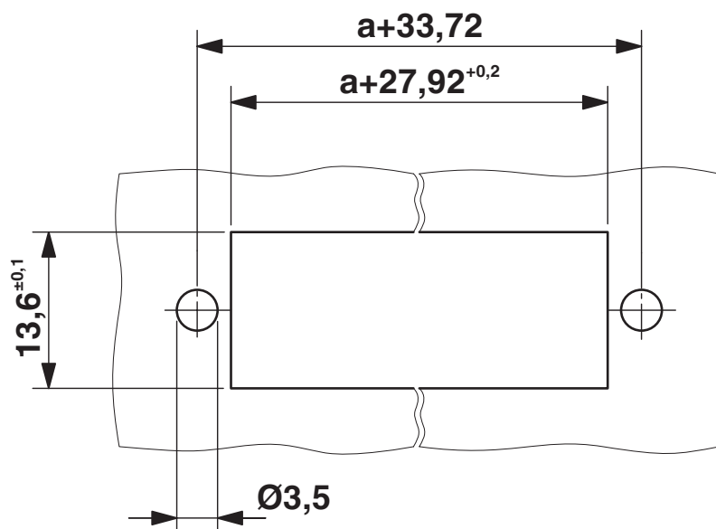
尺寸图
