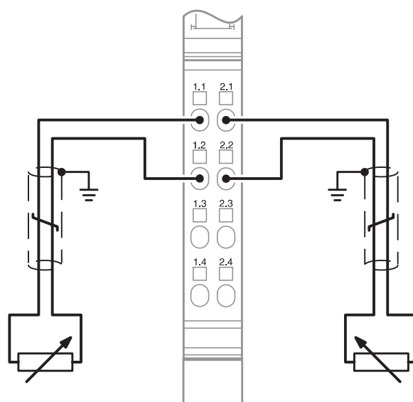
接线图
