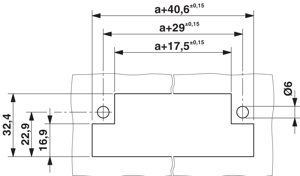
尺寸图
