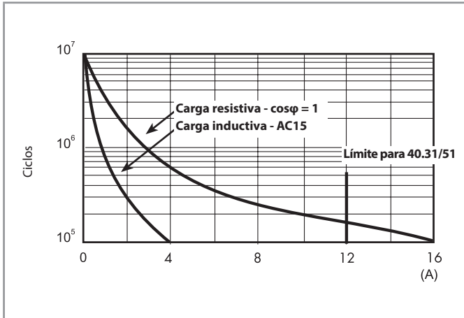
F 40.6 - Vida útil eléctrica (AC) en función de la carga Tipo 40.62
