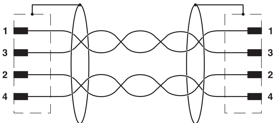
电路图
