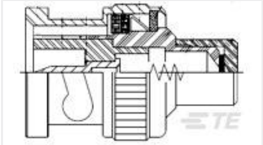
TE Part #1-1337523-0 BNC Plg Term 50Ohm Nickel Pltd
