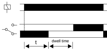
TIMING DIAGRAM DIAGRAMME DES TEMPS ZEITDIAGRAMM
