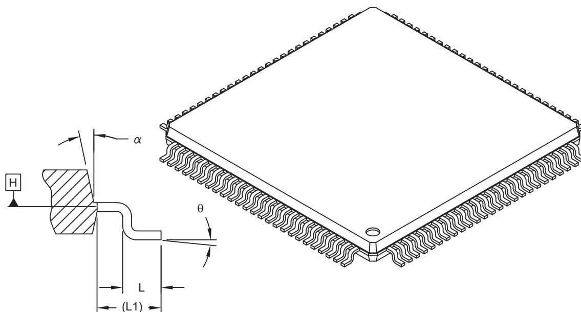
SECTION A-A
