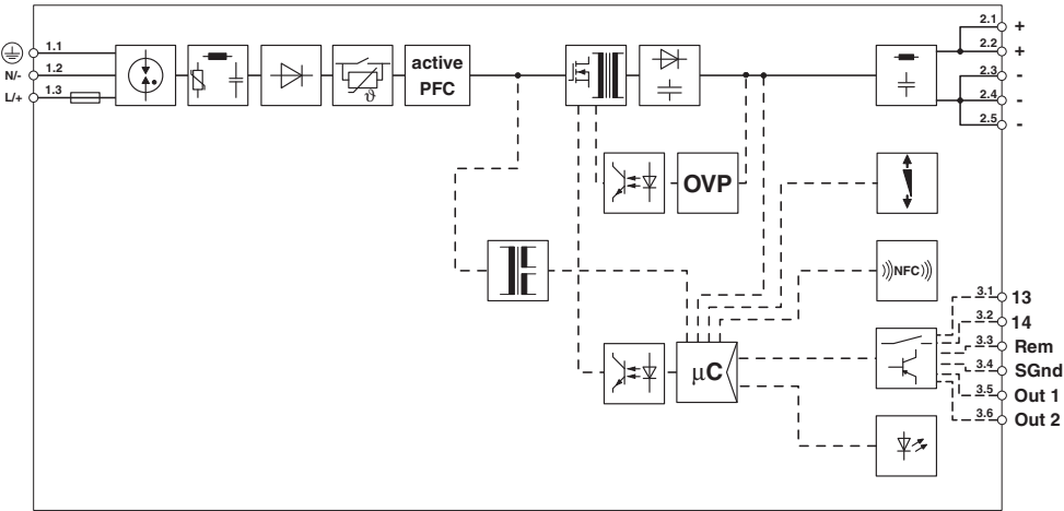
结构框图
