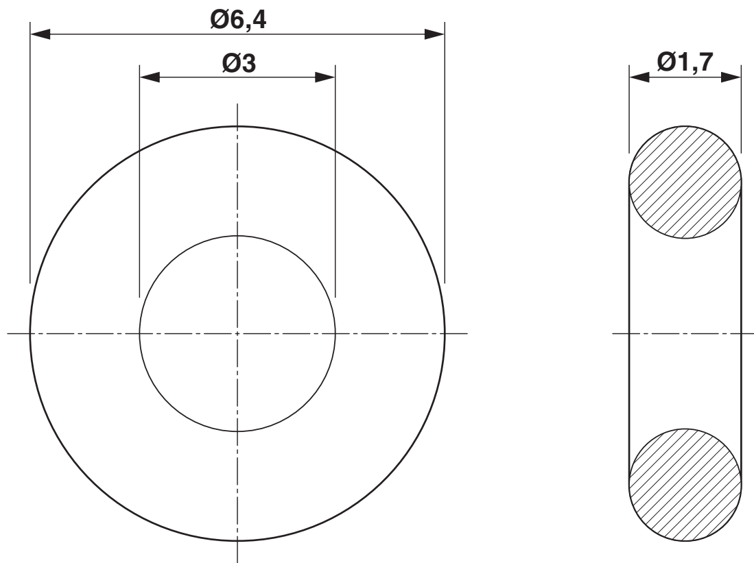
尺寸图
