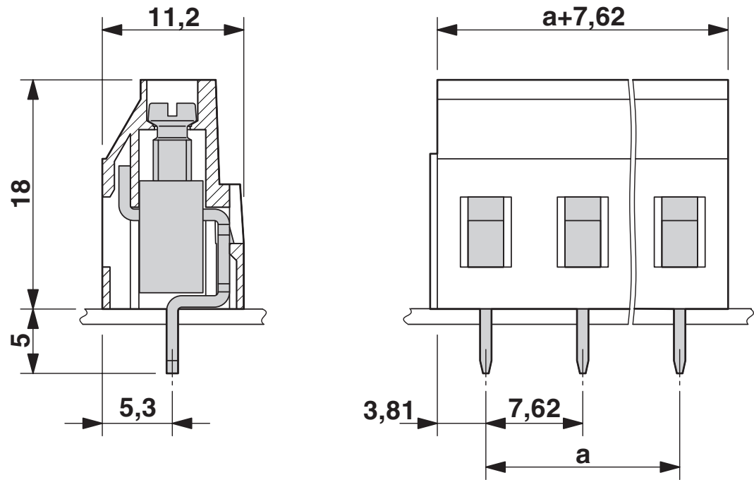
尺寸图
