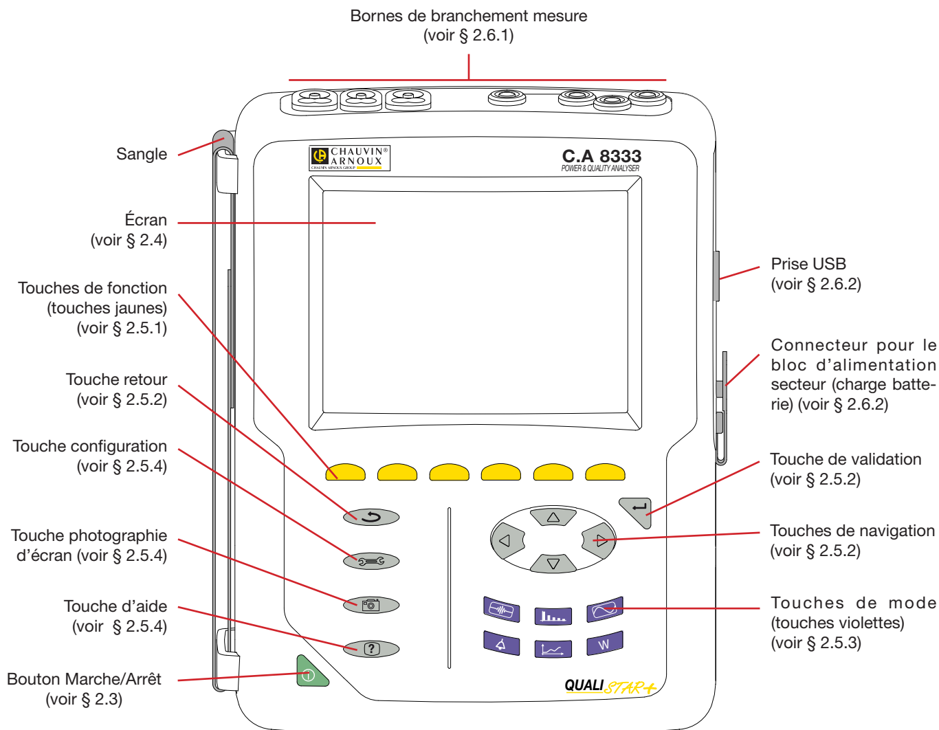
Figure 2 : Vue générale du Qualistar+
