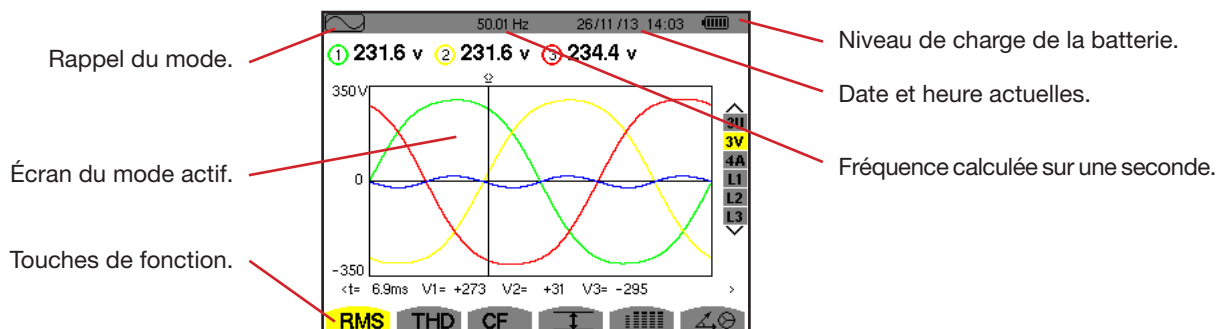
Figure 3 : Exemple d'un écran de visualisation
