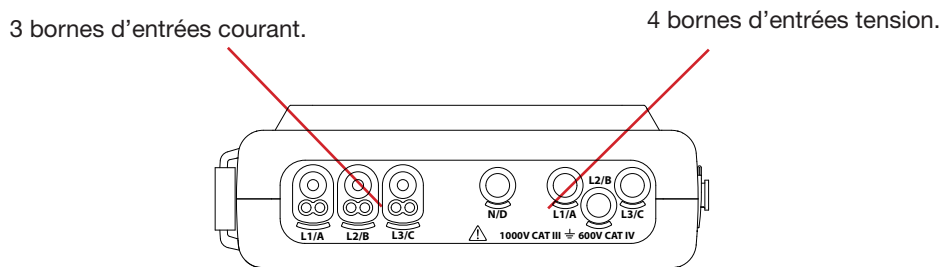
Figure 11 : Les bornes de branchement
