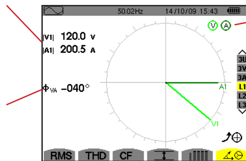
Figure 72 : L'écran d'affichage du diagramme de Fresnel en L1
