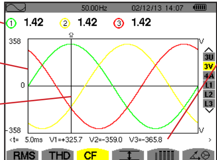
Figure 61 : L'écran d'affichage CF en 3V
