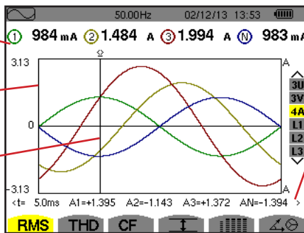
Figure 55 : L'écran d'affichage RMS en 4A
