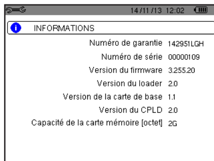
Figure 112 : Le menu Informations
