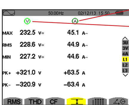
Figure 66 : L'écran d'affichage Max-Min en L1
