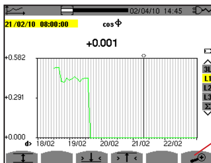
Figure 95 : cos Φ (L1) chargement/calcul des valeurs complet sans MIN-AVG-MAX pour un branchement triphasé avec neutre.
