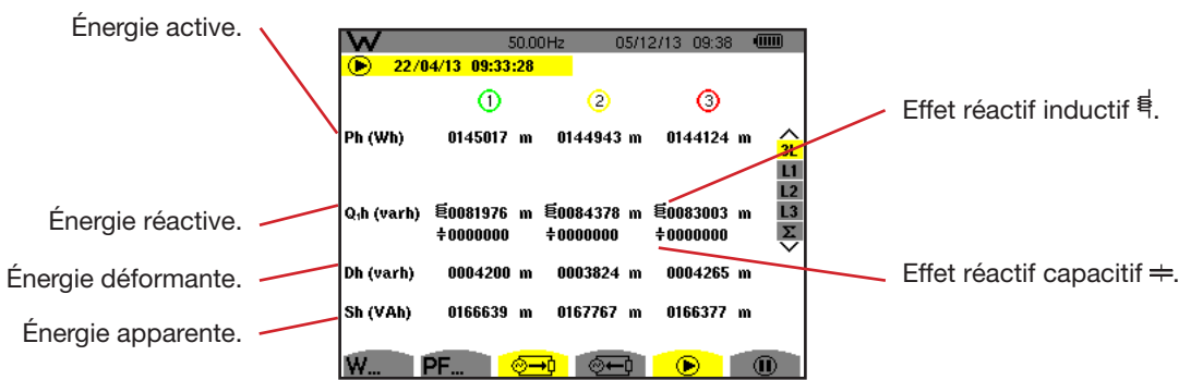
Figure 99 : L'écran d'affichage des énergies consommées en 3L
