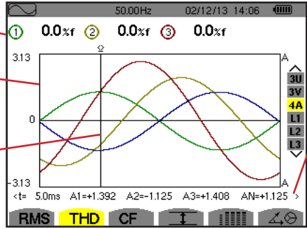
Figure 59 : L'écran d'affichage THD en 4A
