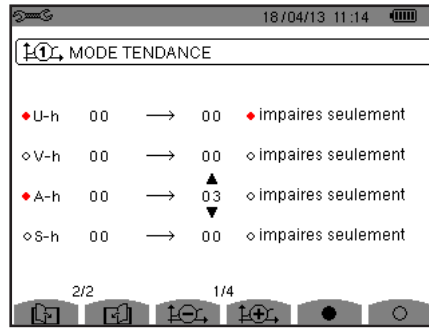
Figure 33 : Le deuxième écran du Mode tendance en cours de modification
