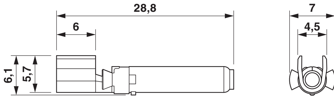
外形寸法
