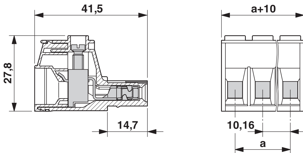
尺寸图
