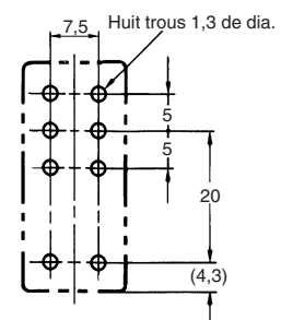
Trous de fixation Huit trous 1,3 de dia.
