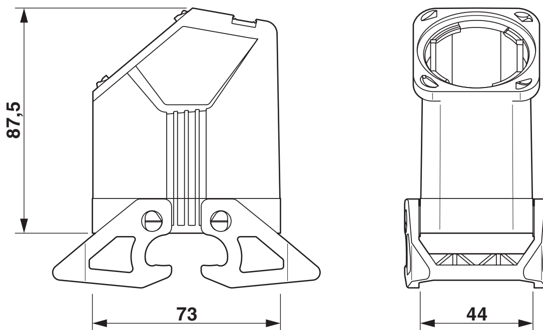
Maßzeichnung
