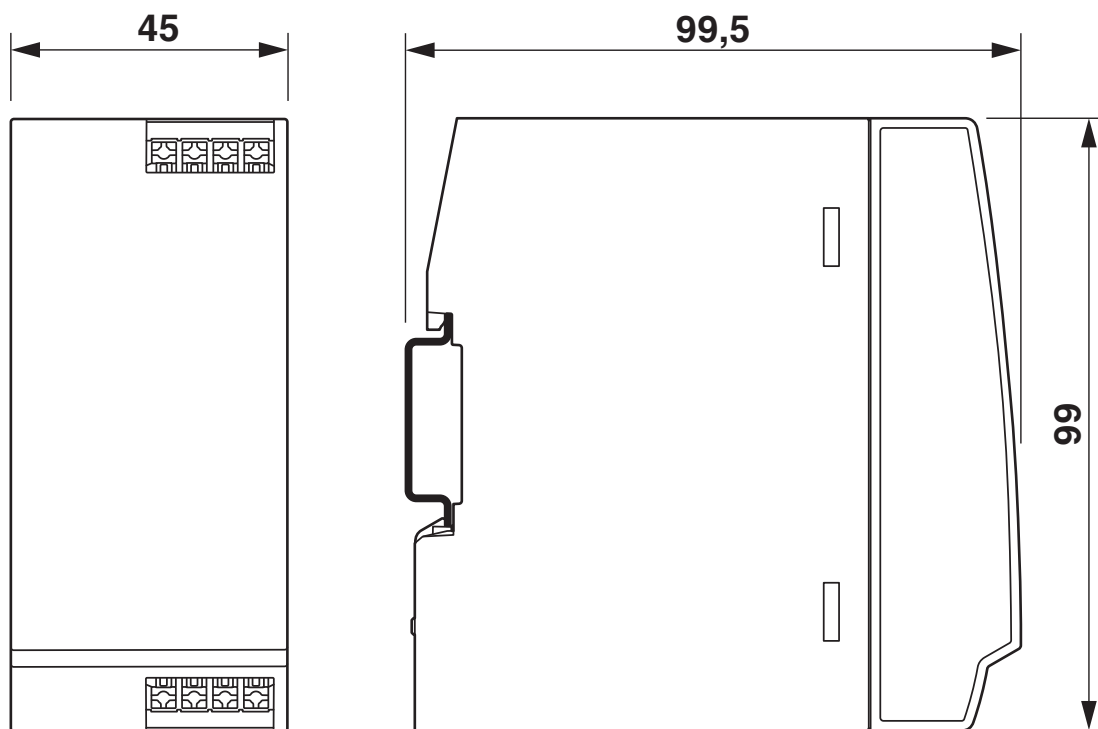
尺寸图
