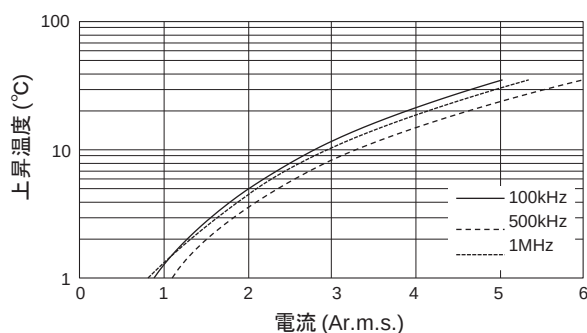
リップル発熱特性
