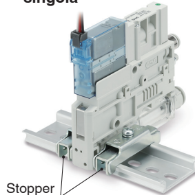
■ Montaggio su guida DIN unità singola
