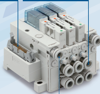
Attacco (PV) di alimentazione pressione pneumatica comune
