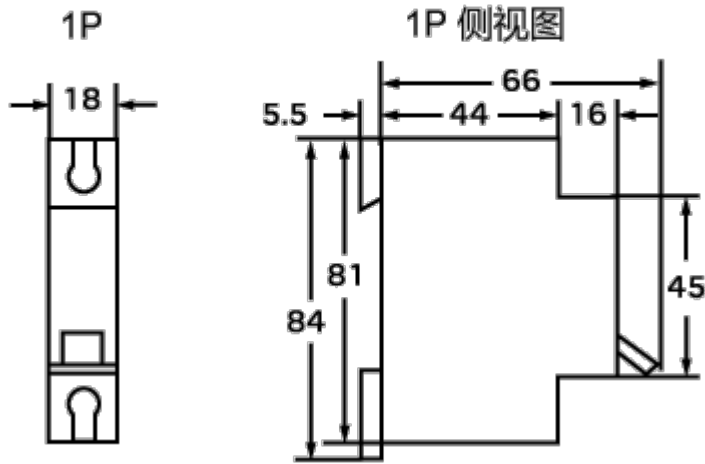
尺寸 (mm)
