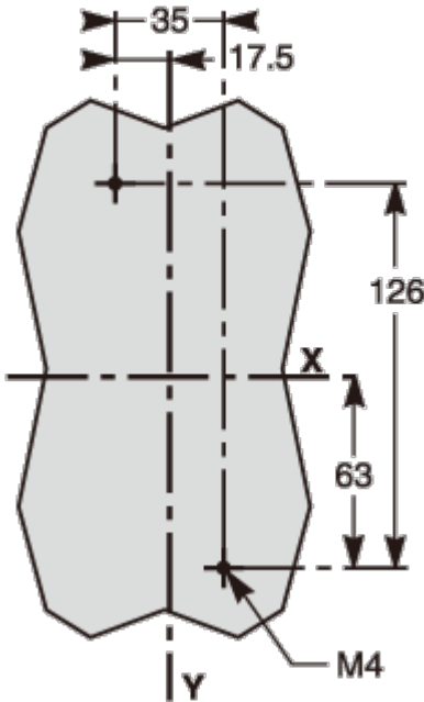
底板安装（3P）
