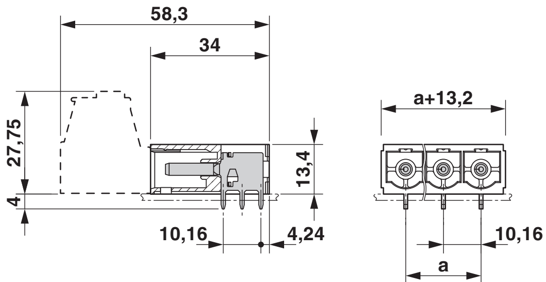
尺寸图
