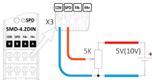
Steuerung mit einem externen Potentiometer
