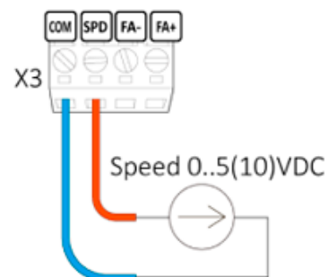
Steuerung mit einer externen Spannung Quelle 0..5V oder 0..10V
