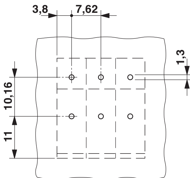
Bohrplan/Lötpadgeometrie
