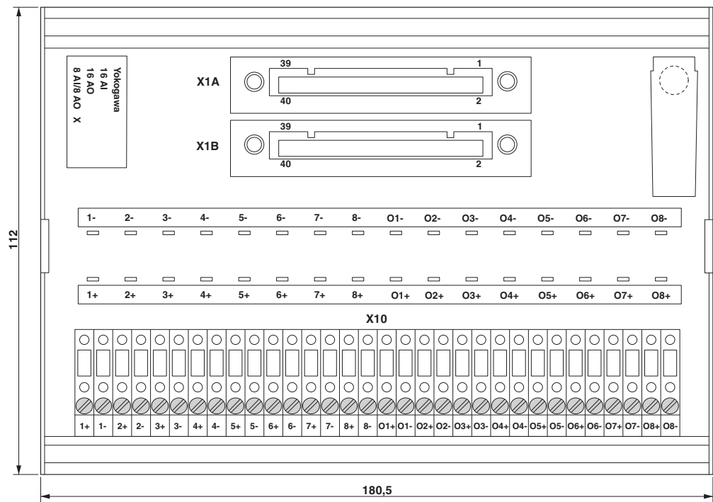
Maßzeichnung
