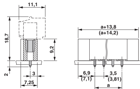
外形寸法
