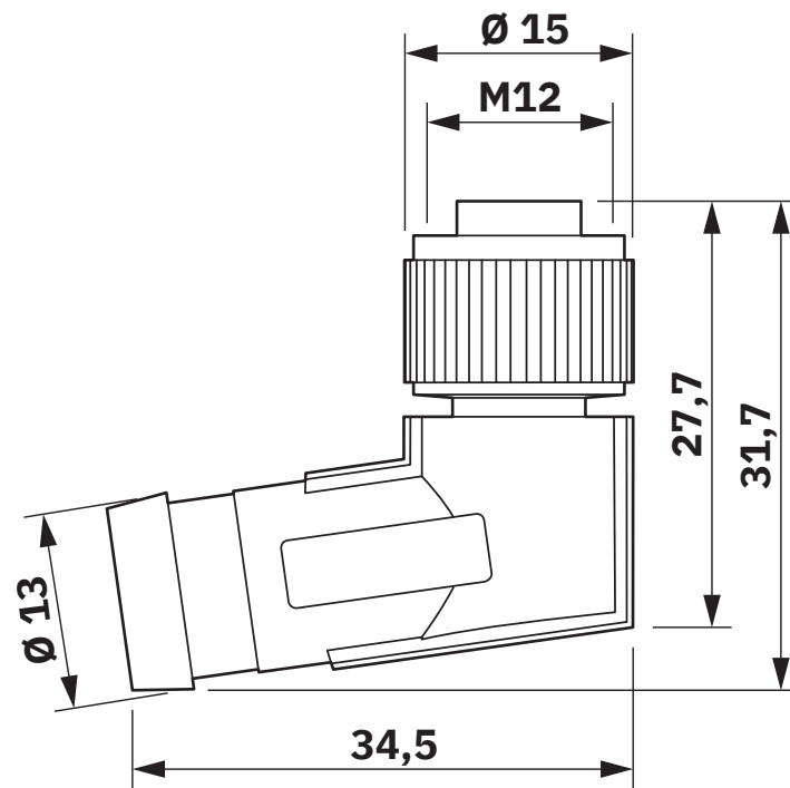
尺寸图
