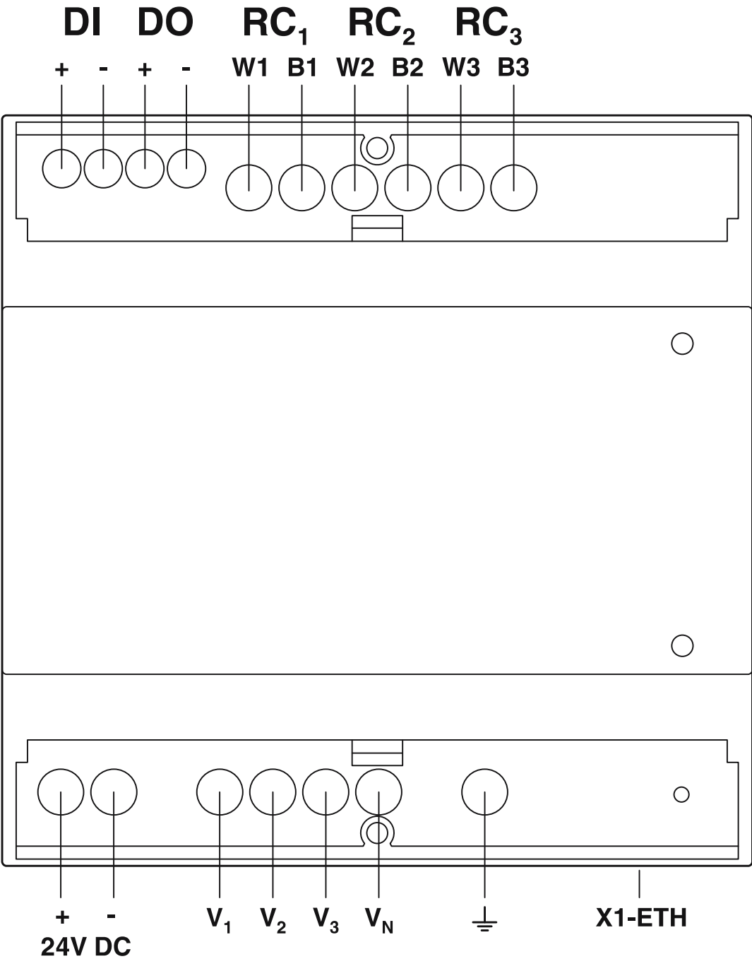
接线图
