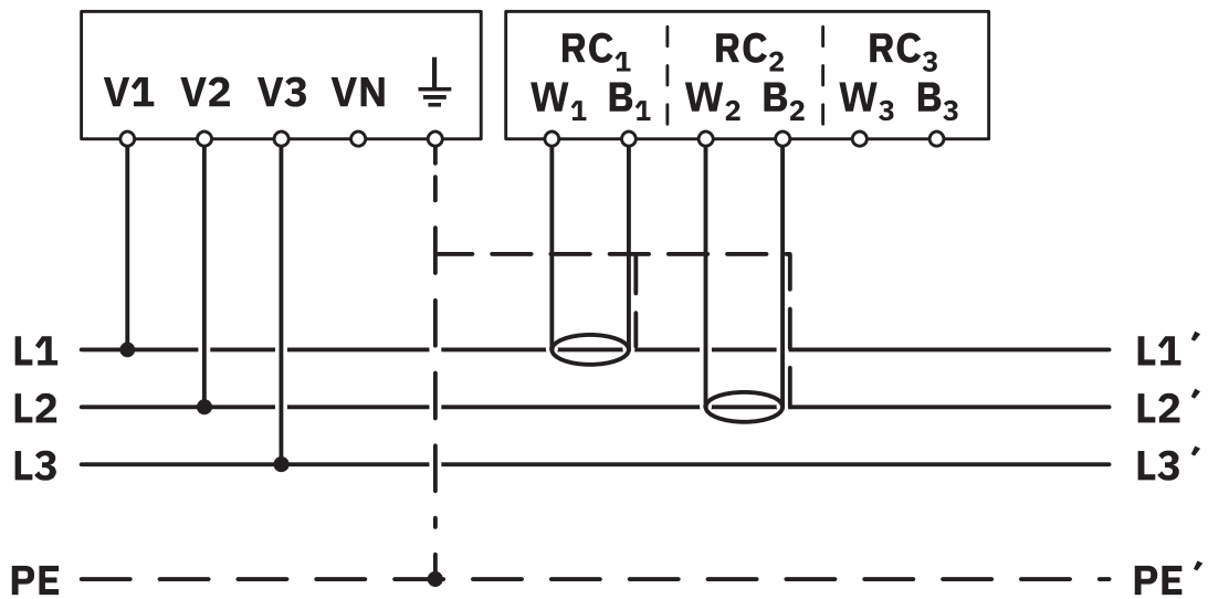
接线图
