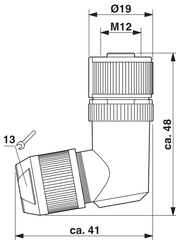
尺寸图
