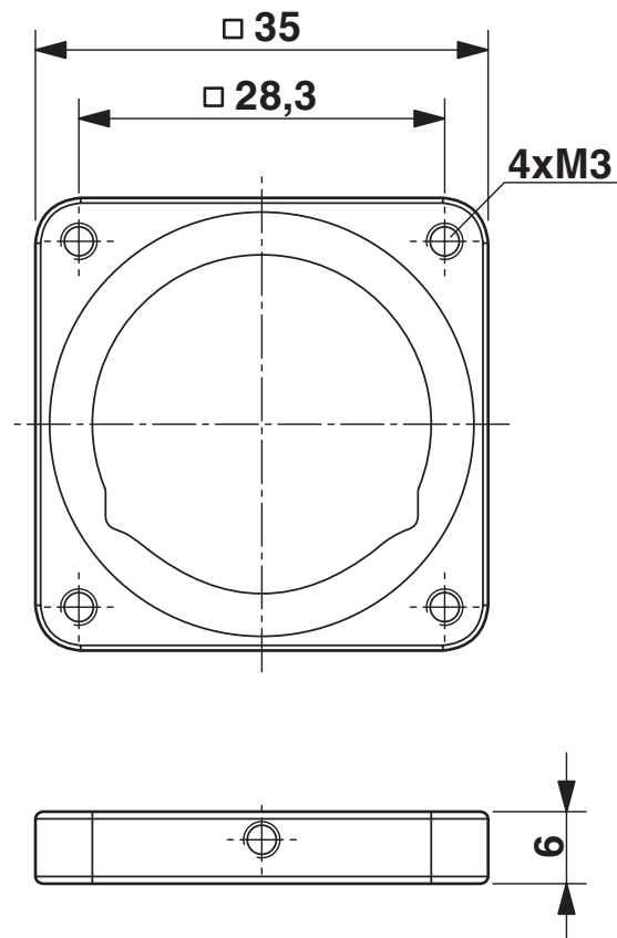
尺寸图
