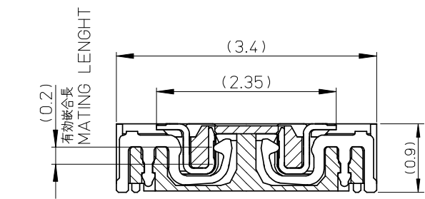
嵌合断面図 (参考) MATED DRAWING
