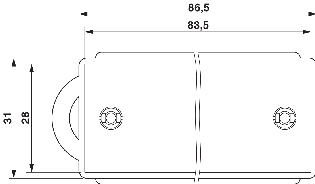
尺寸图
