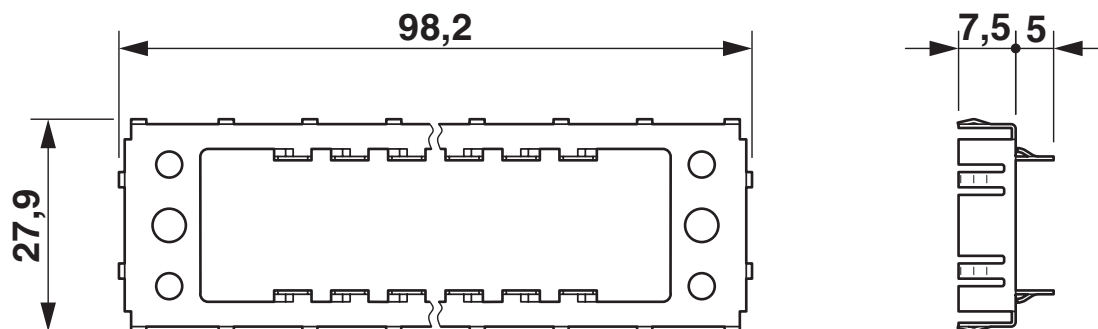
尺寸图
